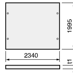
頂版スラブ (H=2500)
