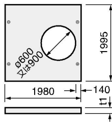
点検用スラブ (H=1000~H2000用)
