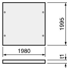
頂版スラブ (H=1000~H2000用)
