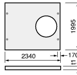
点検用スラブ (H=2500)
