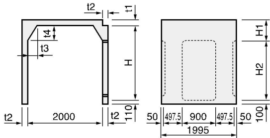
頂版スラブ (H=1000~H2000用)
