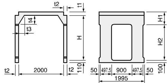
頂版スラブ (H=2500)
